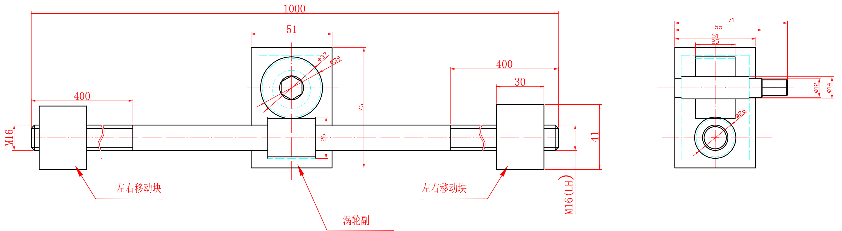
蜗轮蜗杆传动示意图
